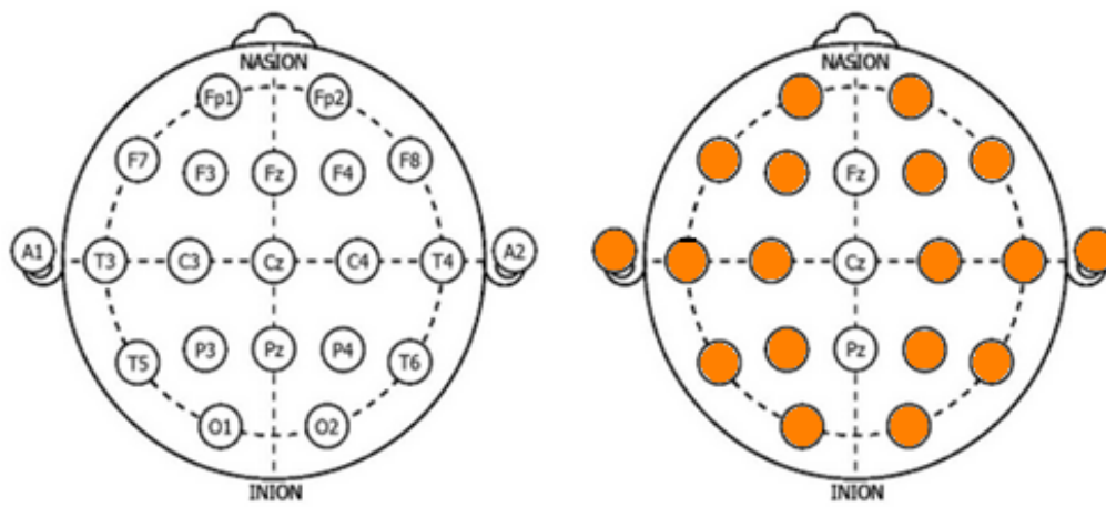
Figura 20 – Posicionamento dos eletrodos.
