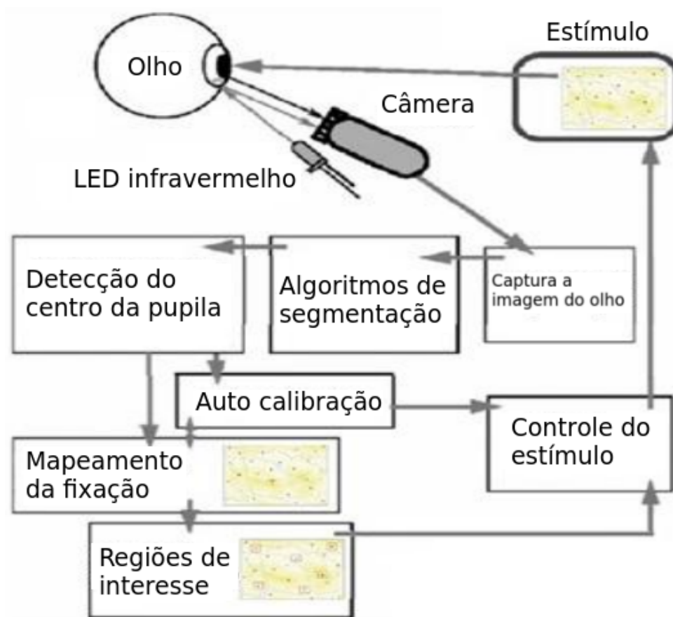
Figura 14 – Diagrama de funcionamento da VOG.
