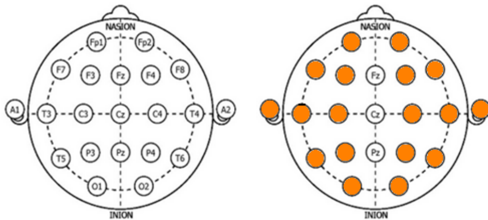
Figura 14 – Posicionamento dos eletrodos.
