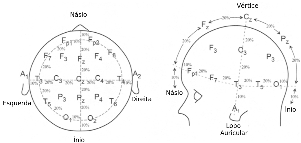
Figura 6 – Posicionamento dos eletrodos no sistema internacional 10-20.
