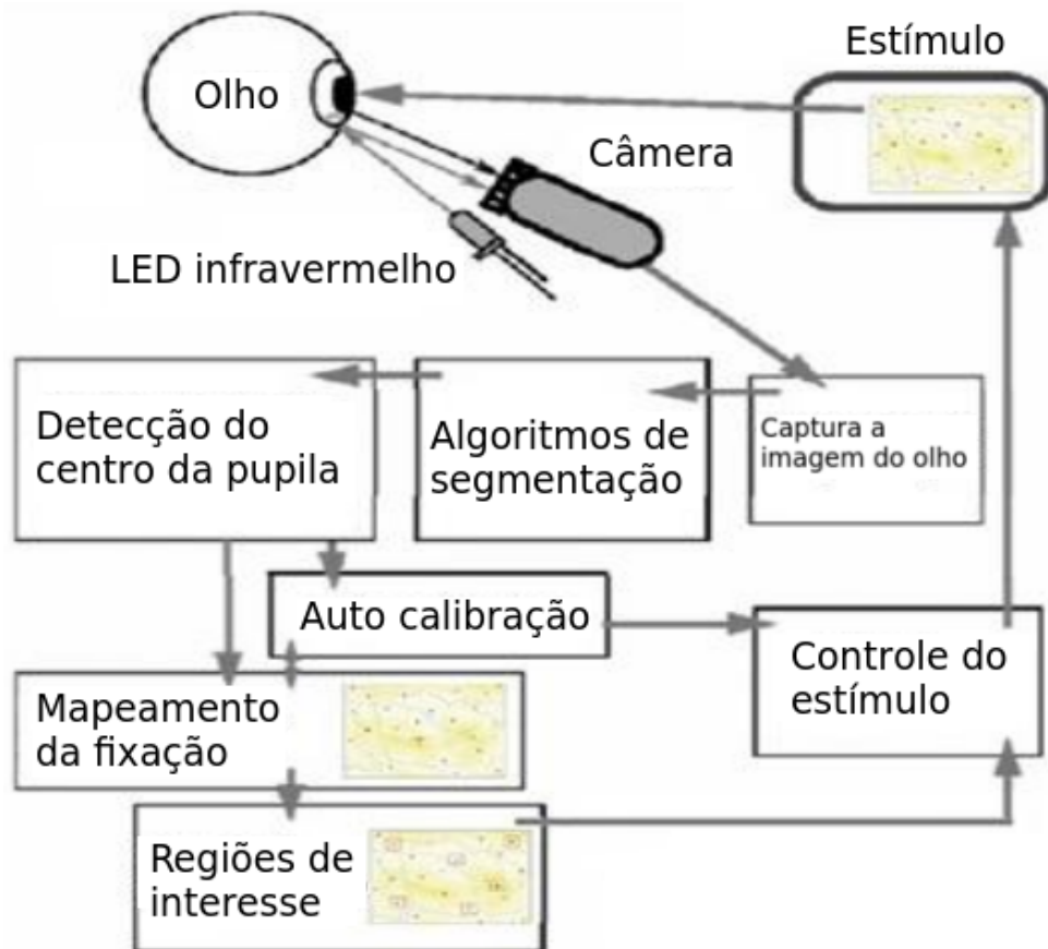
Figura 11 – Diagrama de funcionamento da VOG.
